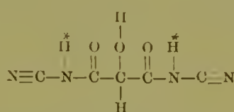
\text{C}_3\text{H}_2\text{O}_3(\text{NH.CN})_2 Tartronyl-Cyanamid (Harnsäure).
